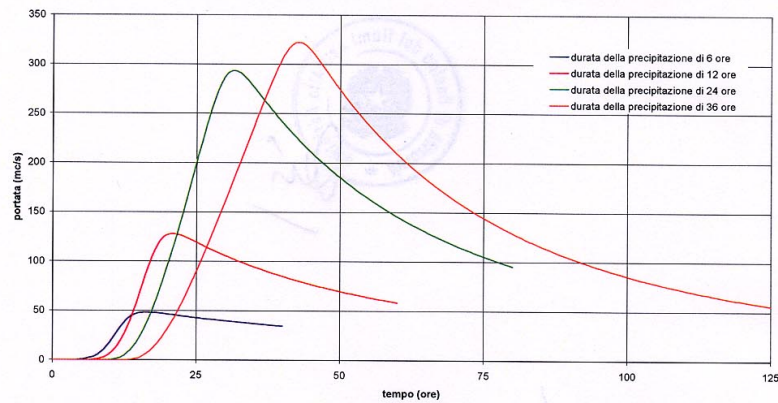
Fiume Livenza a monte di Tremeacque - Onde di piena sintetiche da eventi di pioggia con Tr = 500
