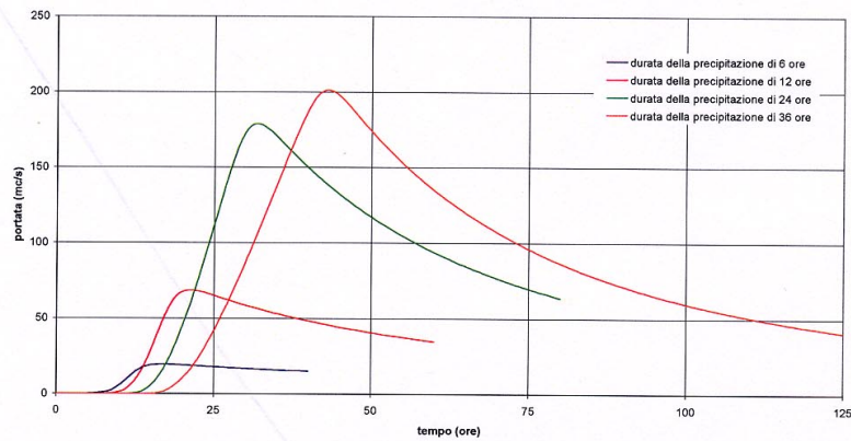
Fiume Livenza a monte di Tremeacque - Onde di piena sintetiche da eventi di pioggia con Tr = 100
