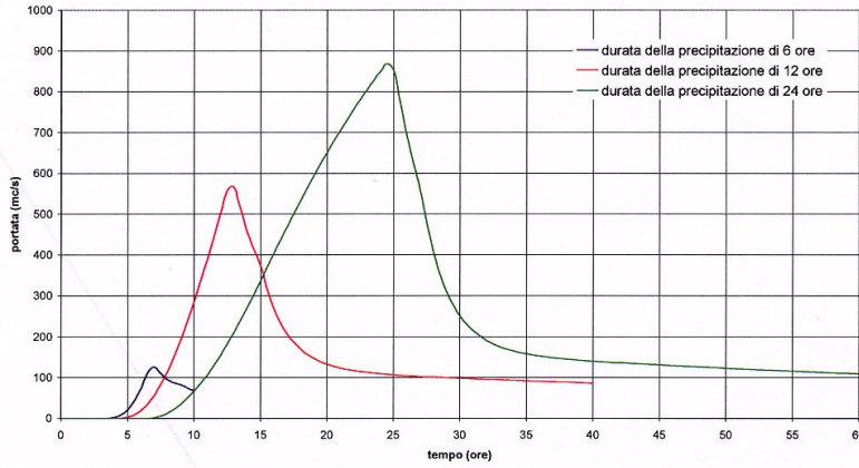
Torrente Cellina a Ravedis - Onde di piena sintetiche da eventi di pioggia con Tr = 100
