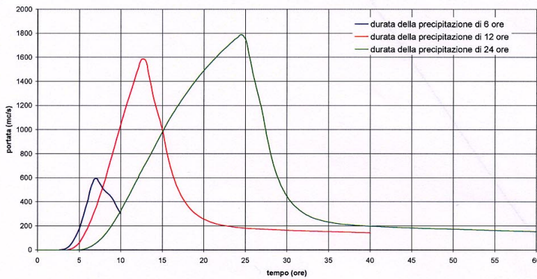
Figura 12.3: Idrogrammi di piena sintetica derivanti dall'applicazione del modello afflussi-deflussi corrispondentemente a prefissate durate di precipitazione e tempo di ritorno, alla sezione di Ravedis, sul Cellina
