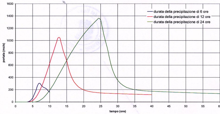
Torrente Cellina a Ravedis - Onde di piena sintetiche da eventi di pioggia con Tr = 500
