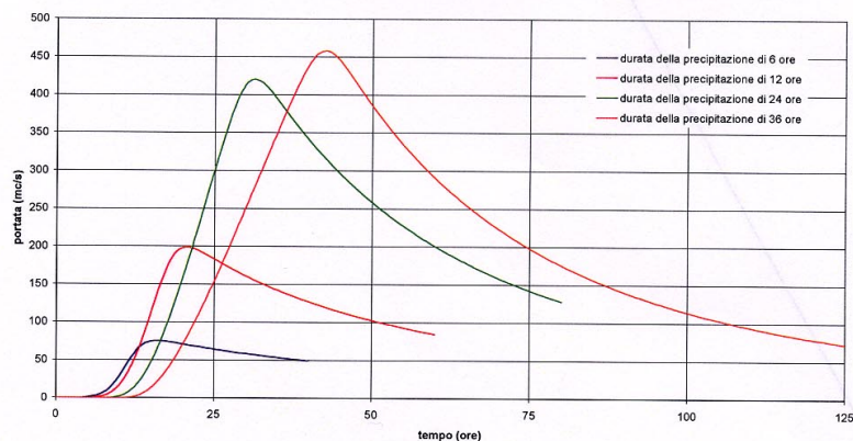
Figura 12.6: Idrogrammi di piena sintetica del fiume Livenza derivanti dall'applicazione del modello afflussi-deflussi corrispondentemente a prefissate durate di precipitazione e tempo di ritorno, alla sezione a monte di Tremeacque
